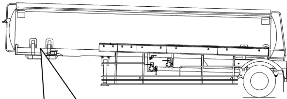
シリアル番号銘板 (フロントフレーム左舷側面)
