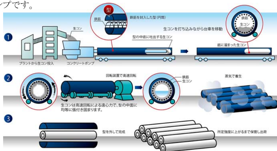
コンクリート二次製品製造フロー図 (例)
