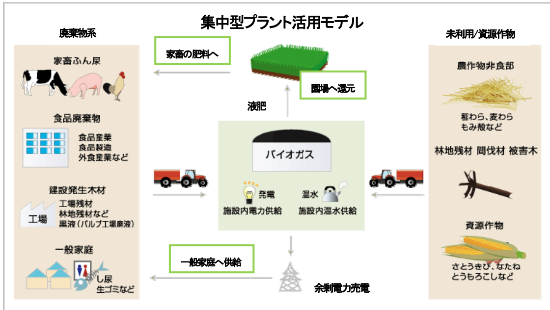
【バイオガスプラントフロー図】
